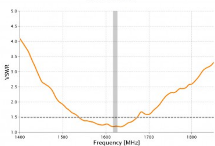
65000 VSWR
